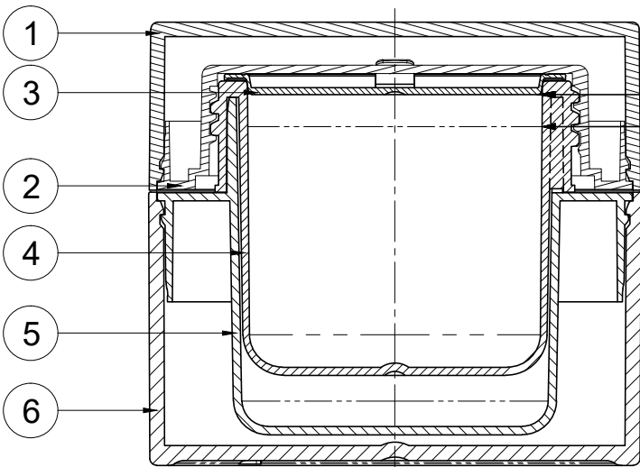
SEC A-A
